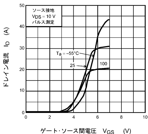
図 8.3 I_D - V_{GS}
