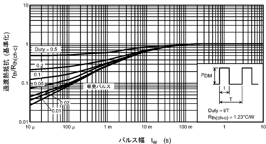
図 8.13 r_{th}/R_{th(ch-c)} - t_w (最大値 (保証値))
