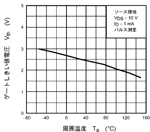
図 8.10 V_{th} - T_a
