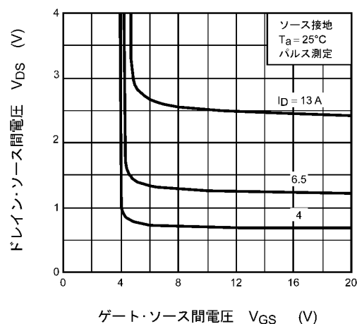
図 8.4 V_{DS} - V_{GS}
