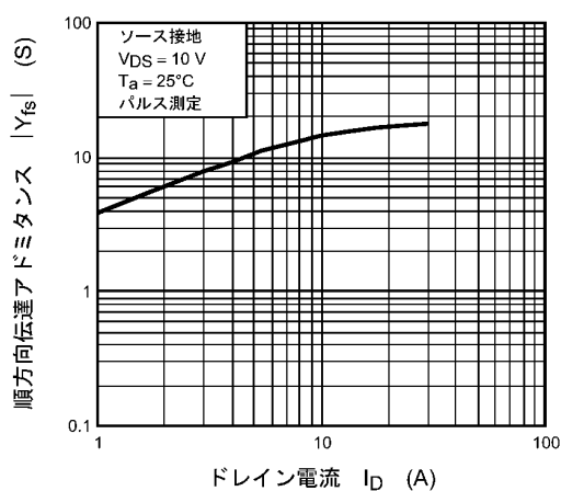
図 8.5 |Y_{fs}| - I_D
