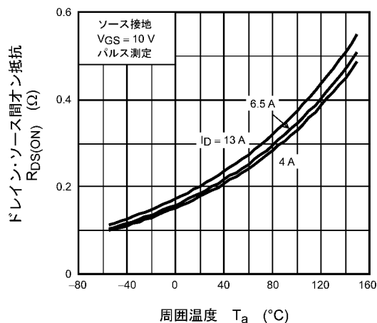
図 8.7 R_{DS(ON)} - T_a
