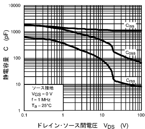
図 8.9 C - V_{DS}
