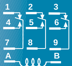
3PDT
