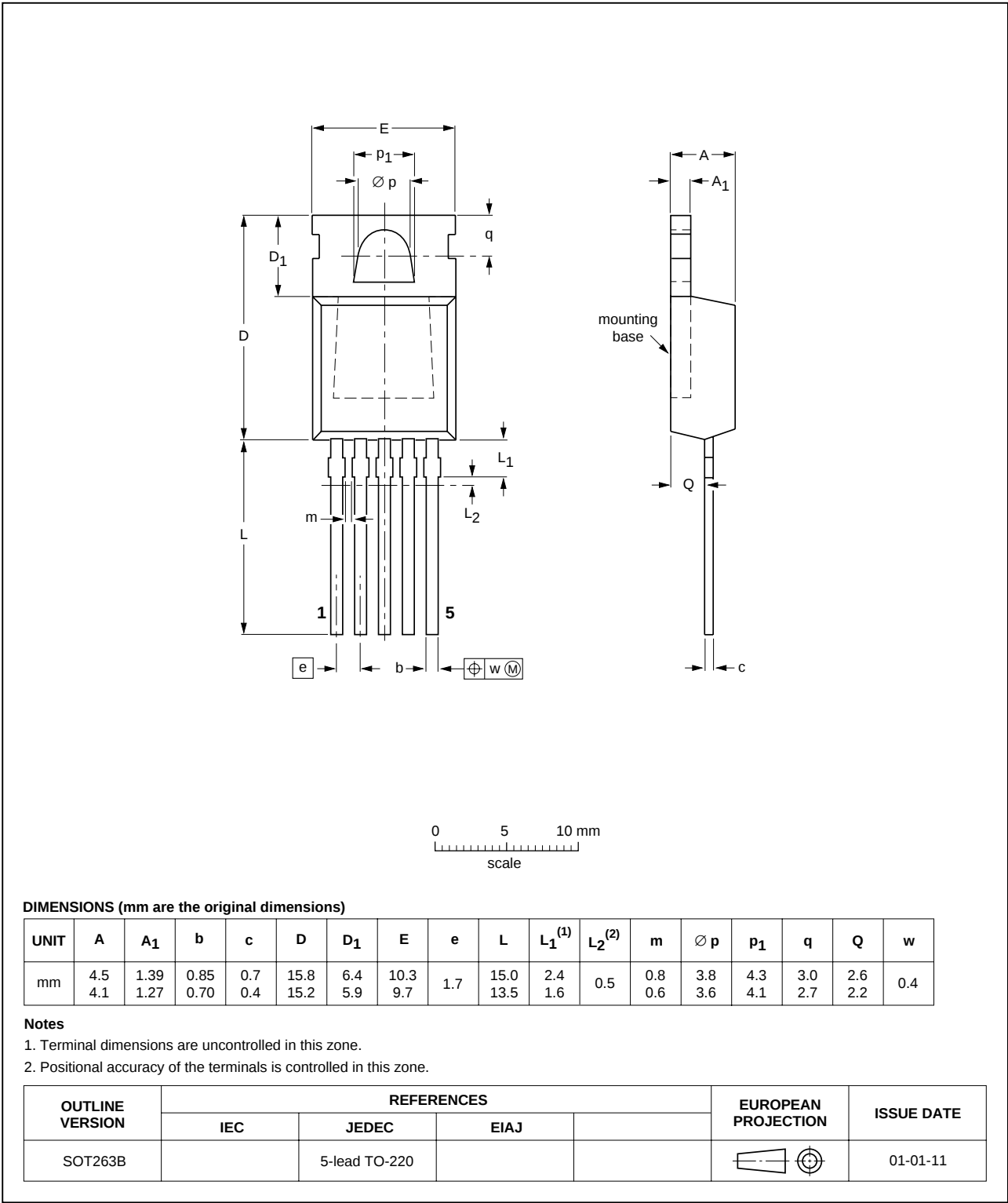
Fig 19. SOT263B.
