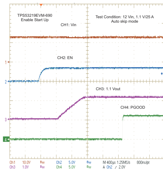
Figure 7-7. Enable Turn-On
