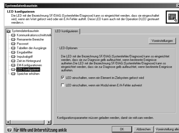
Bild 4-28 Diagnose-LED
