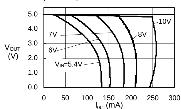
S-817B50A(Ta=25°C)
