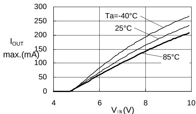
S-817B50A
