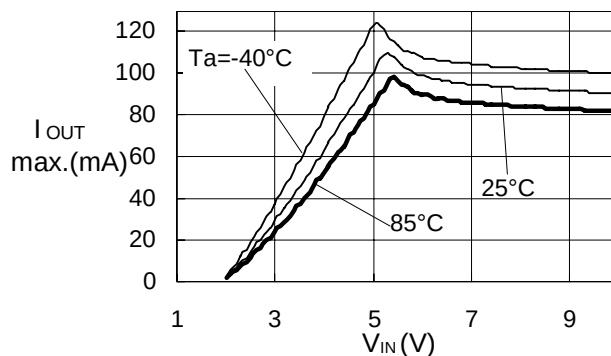
S-817A50A
