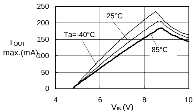
S-817A50A
