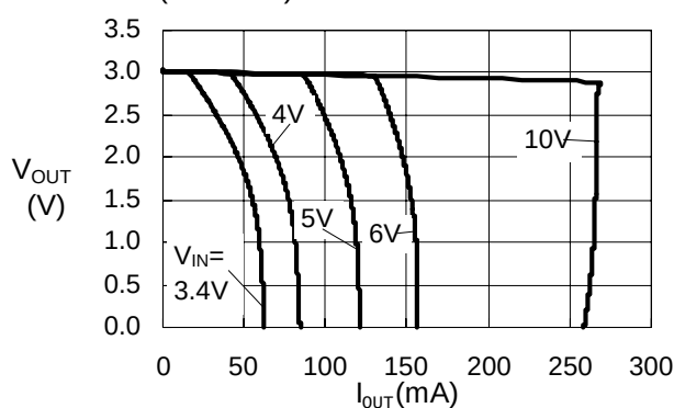
S-817B30A(Ta=25°C)
