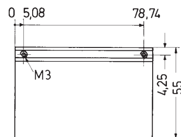
Mögliche Ausführung mit 5xM3
