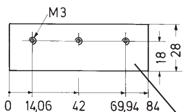
Abb. Montageseite
