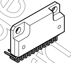
HZIP23-P-1.27F (LBR)
