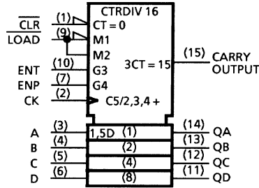
TC74ACT161
