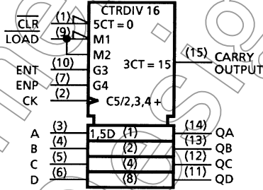
TC74ACT163
