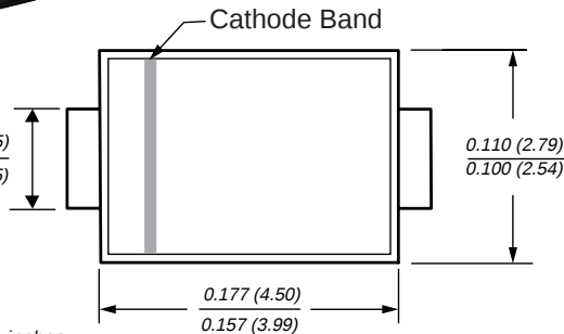
DO-214AC (SMA)
