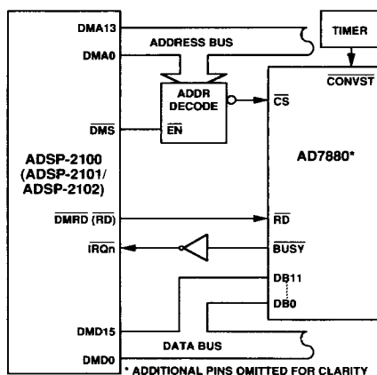
Figure 15. AD7880-ADSP-2100 (ADSP-2101/ADSP-2102) Interface
