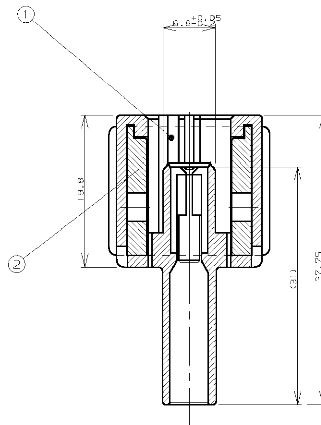
SCHNITT A-A
