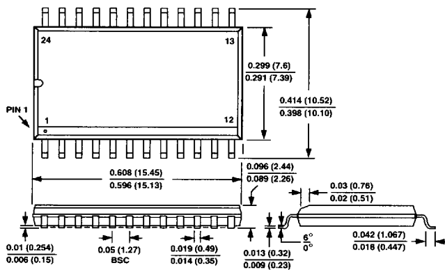
SOIC (R-24)
