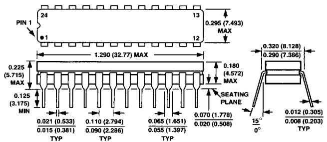
Cerdip (Q-24)
