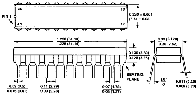
Plastic (N-24)
