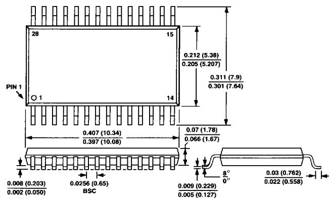
SSOP (RS-28)
