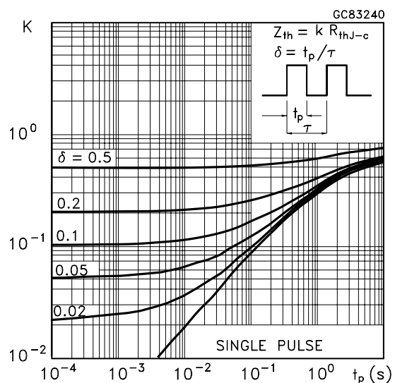
Thermal Impedance
