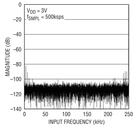
248kHz Sine Wave 8192 FFT Plot
