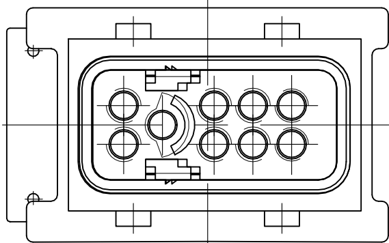
Vorraststellung
