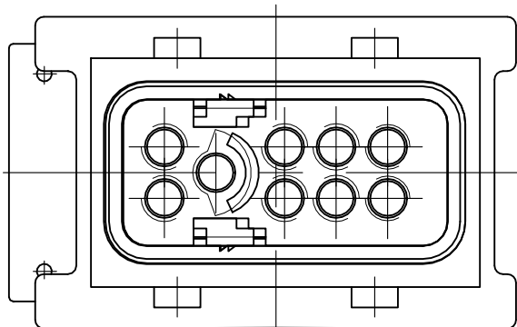
Vorraststellung
