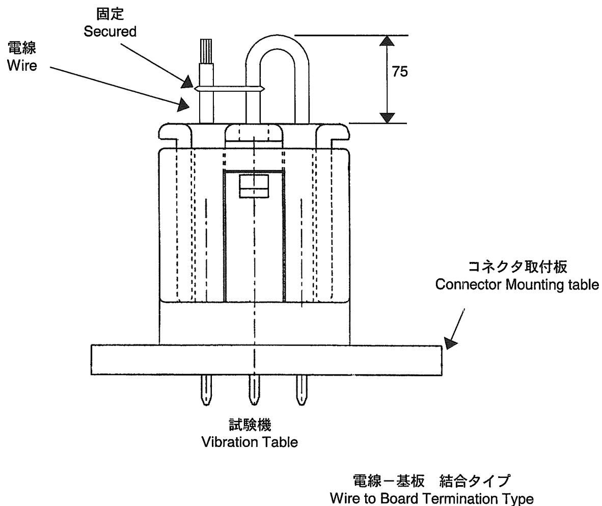
Fig. 7 低周波振動試験及び衝撃試験のコネクタ取付方法 Connector Mounting Methods of Low Frequency Vibration & Physical Shock Tests
