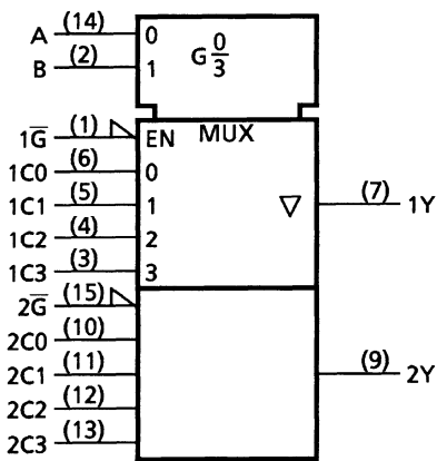
TC74HC253A
