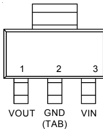
SOT-223
