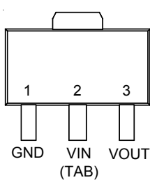
SOT-89 (L-Type)
