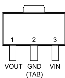
SOT-89
