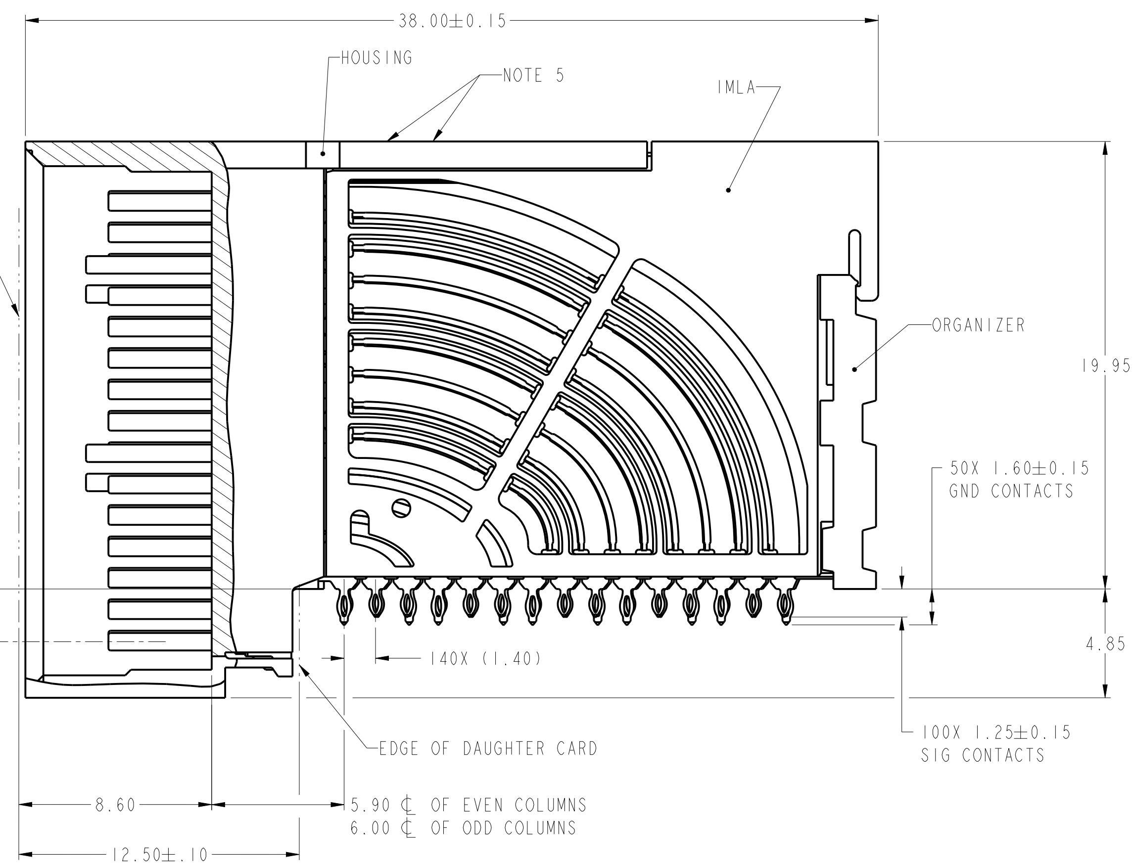
SECTION AA-AA
