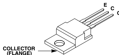
JEDEC TO-220AB
