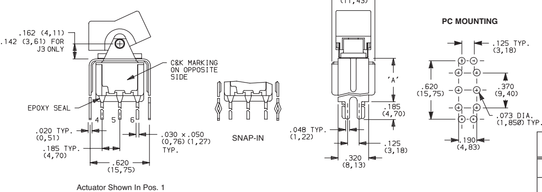
7201J1_BE2 DPDT
