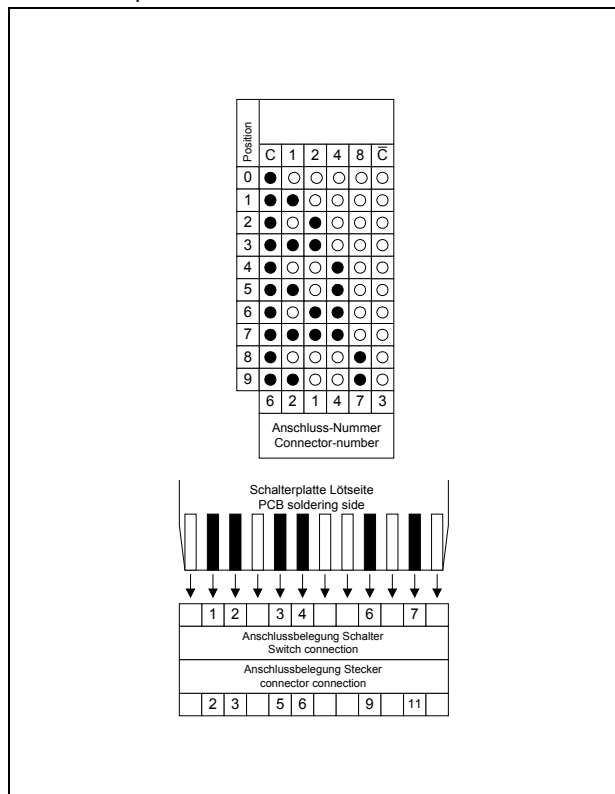
Code 140 BCD + 2 inputs
