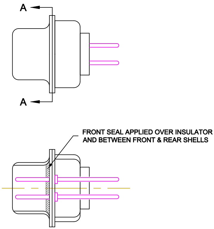
DETAIL A-A
