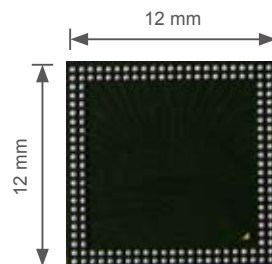
■ LPDDR2_168WFBGA
