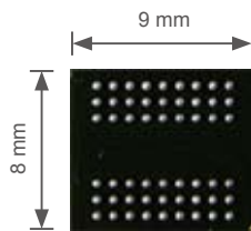
■ SDRx16_54BGA
