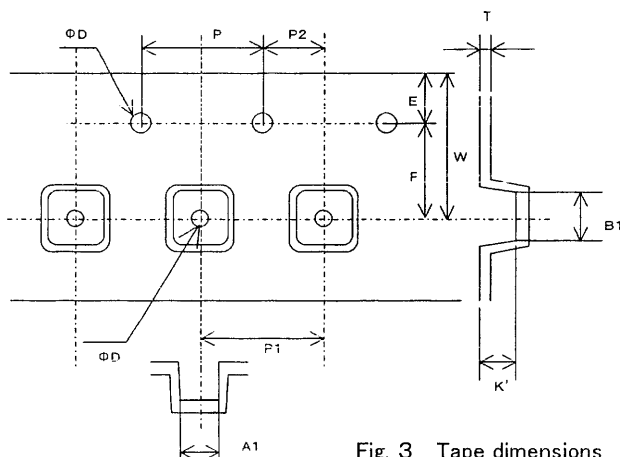
Fig. 3 Tape dimensions
