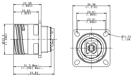
USBF TV 2 XX
