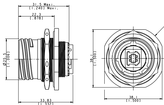
USBF TV 7 XX
