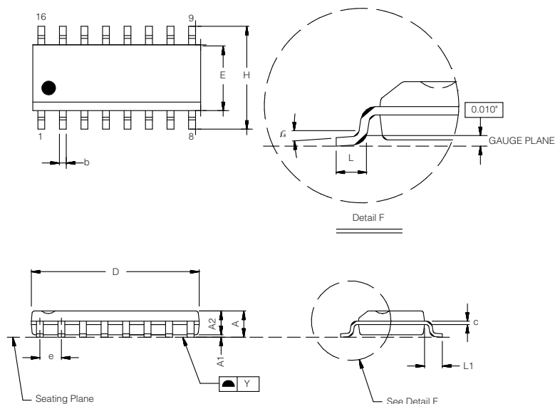
16 PIN SOIC
