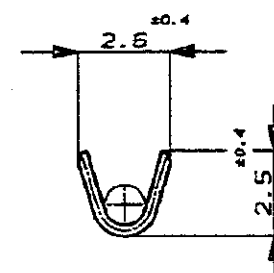
断面 A-A SECT.
