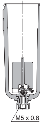
Float type auto drain (N.C.)
