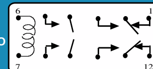
219BBXP DPDT+2 NO
