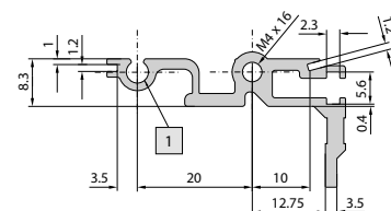
1 Core hole M4
