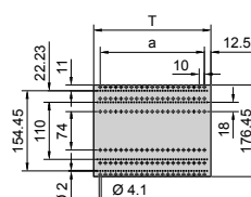
7 U (6 U + 2 x ½ U)
