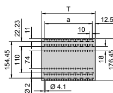
7 U (6 U + 2 x ½ U)
