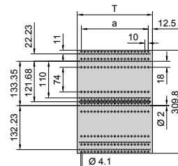
7 U (6 U + 2 x ½ U)
