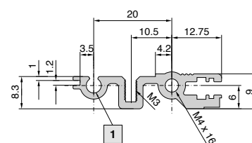
1 Core hole M4
