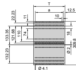
7 U (6 U + 2 x ½ U)
