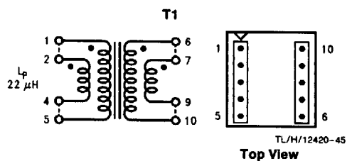
FIGURE 29. Schott 67141450
