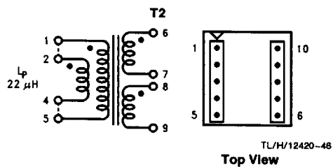
FIGURE 30. Schott 67140860
