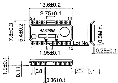
HSOP25 (Unit:mm)
