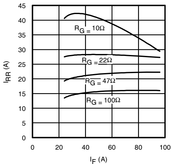
Fig. 17 - Typ. Diode I_{\text{RR}} vs. I_{\text{F}}
