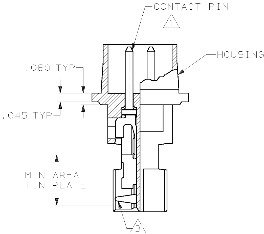
SECTION A-A
