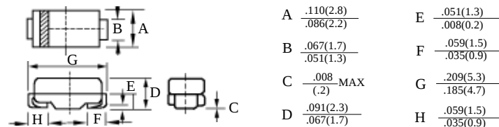
DO – 214AC
