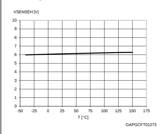
Figure 34: Vsenseh vs. Tcase
