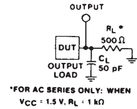
Fig. 6 - Test circuit.
