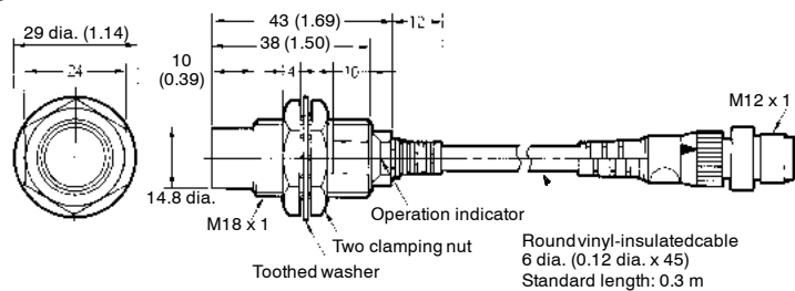
Fig. 22: E2E-X14MD1-M1GJ-N
