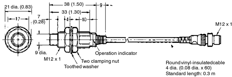
Fig. 21: E2E-X7D1-M1GJ-N E2E-X7D1-M1J-T-N
