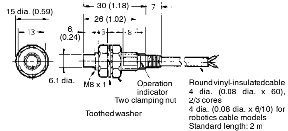
Fig. 4: E2E-X8MD□-N
