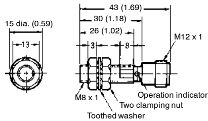
Fig. 9: E2E-X2D□-M1G-N
