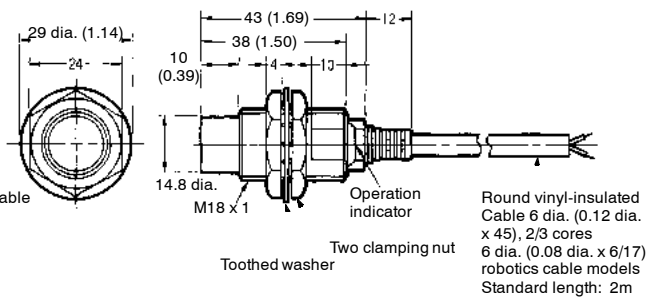
Fig. 6: E2E-X14MD□
