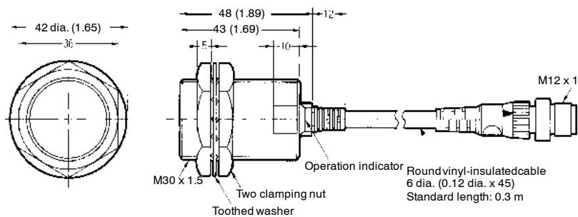
Fig. 24: E2E-X20MD1-M1GJ-N
