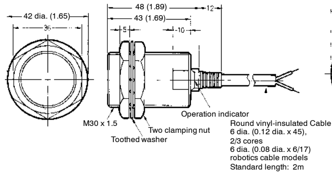
Fig. 7: E2E-X10D□-N
