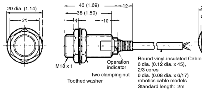
Fig. 5: E2E-X7D□-N
