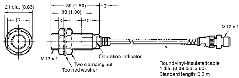
Fig. 20: E2E-X8MD1-M1GJ-N
