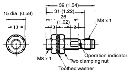
Fig. 17: E2E-X2D□-M3G
