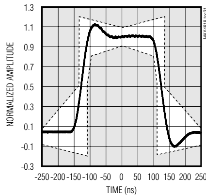
E1 (75Ω) PULSE TEMPLATE TEST
