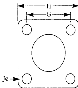
Universal Flange Receptacle
