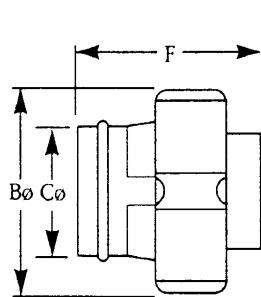
Inline Receptacle
