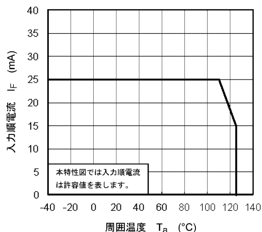
図 12.2.2 I_F - T_a
