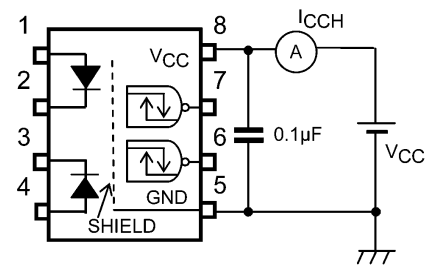
図 12.1.4 ICCH測定回路
