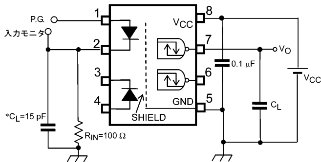
図 12.1.5 伝搬遅延時間測定回路, 波形
