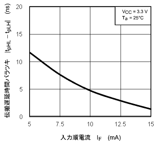
図 12.2.16 |t_{pHL} - t_{pLH}| - I_F
