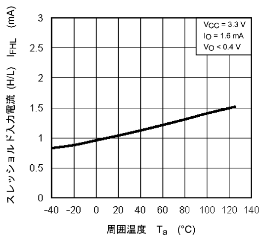
図 12.2.8 I_{FHL} - T_a
