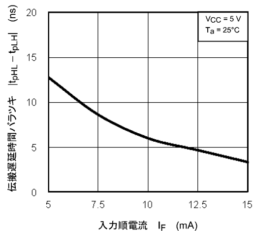
図 12.2.14 |t_{pHL} - t_{pLH}| - I_F
