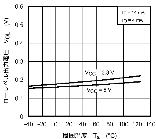
図 12.2.3 V_{OL} - T_a
