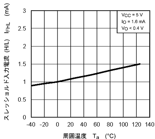
図 12.2.7 I_{FHL} - T_a
