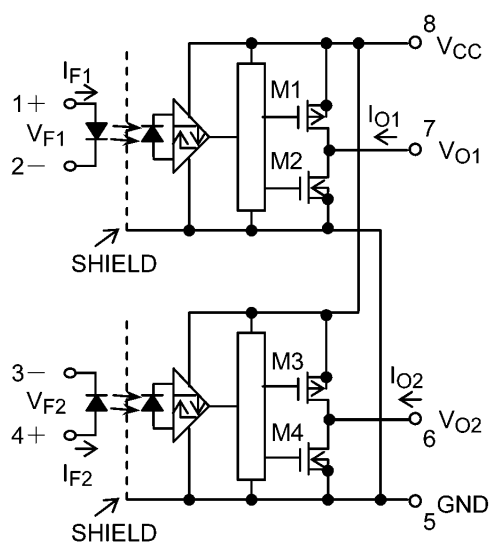
図 5.1 内部回路構成
