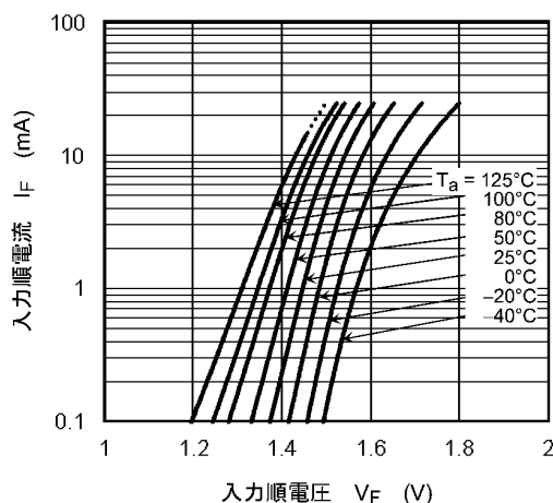
図 12.2.1 I_F - V_F
