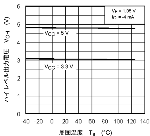
図 12.2.4 V_{OH} - T_a
