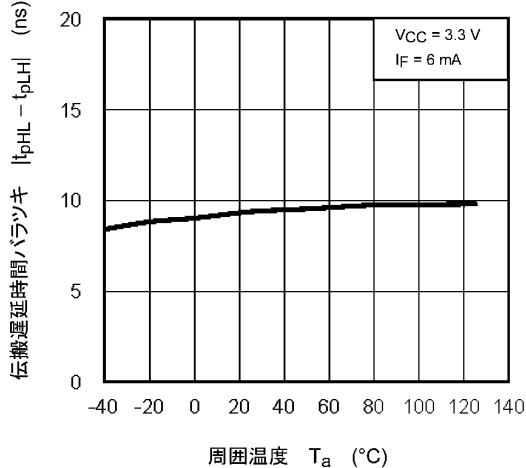
図 12.2.12 |t_{pHL} - t_{pLH}| - T_a
