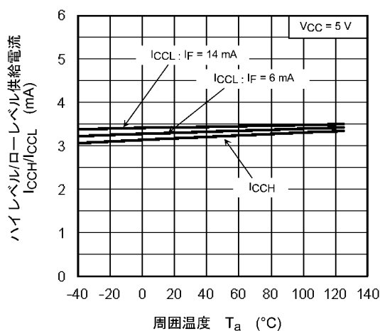
図 12.2.5 I_{CH} / I_{CCL} - T_a
