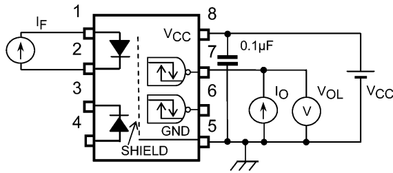
図 12.1.1 VOL測定回路
