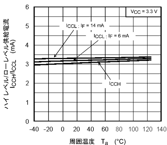
図 12.2.6 I_{CH} / I_{CCL} - T_a
