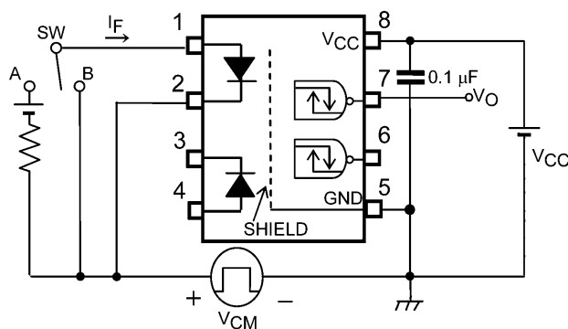
図 12.1.6 コモンモードノイズ除去電圧測定回路, 波形
