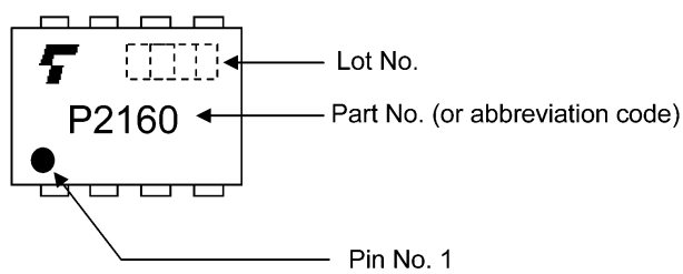
図 15.1 現品表示
