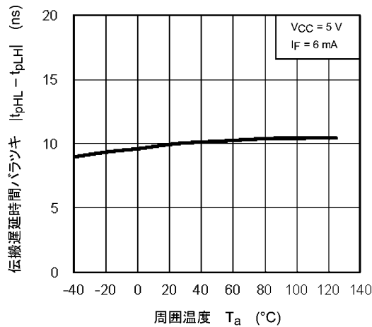
図 12.2.10 |t_{pHL} - t_{pLH}| - T_a
