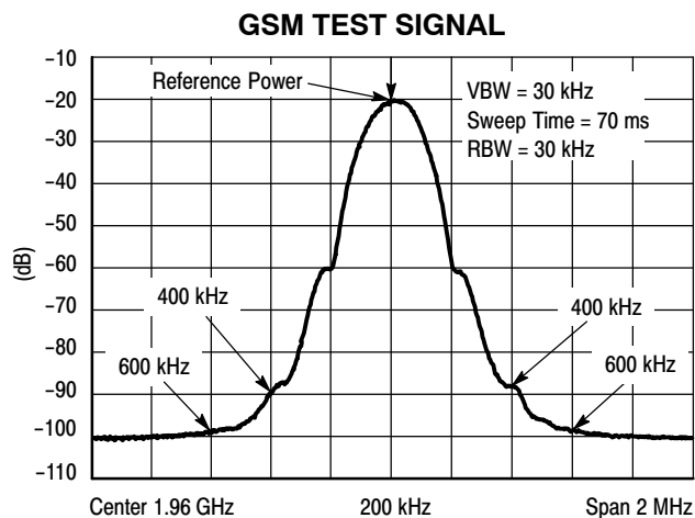
Figure 19. EDGE Spectrum
