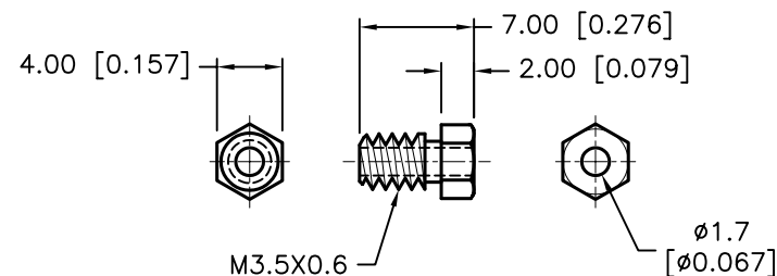
INTERNAL STUD
