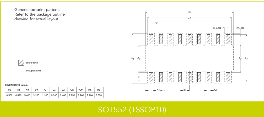
SOT552 (TSSOP10)
