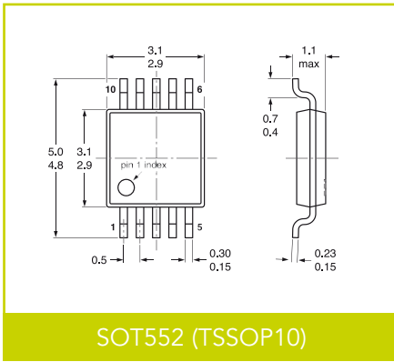
SOT552 (TSSOP10)
