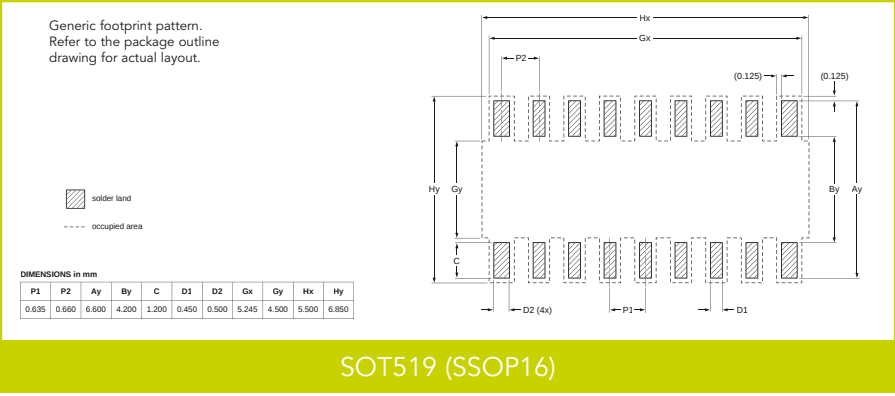
SOT519 (SSOP16)
