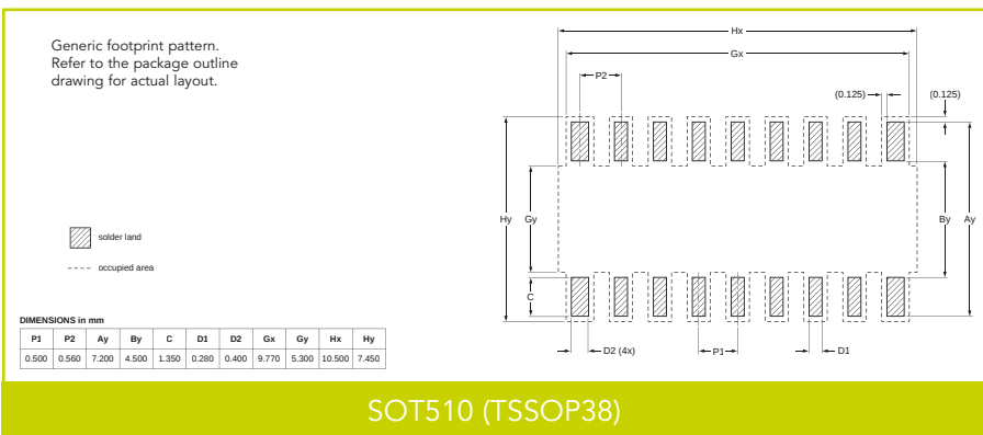
SOT510 (TSSOP38)
