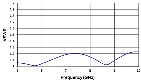
VSWR (5-10 GHz)
