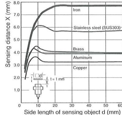
E2A-M18□S08
