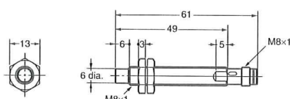
E2A-S08LN04-M5-□□
