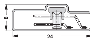
SL 17 SMD ... B SM
