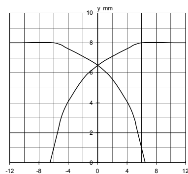
Response characteristics/Ansprechkennlinie:
